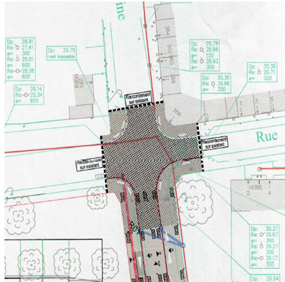
Plateau surélevé avec priorité à droite
