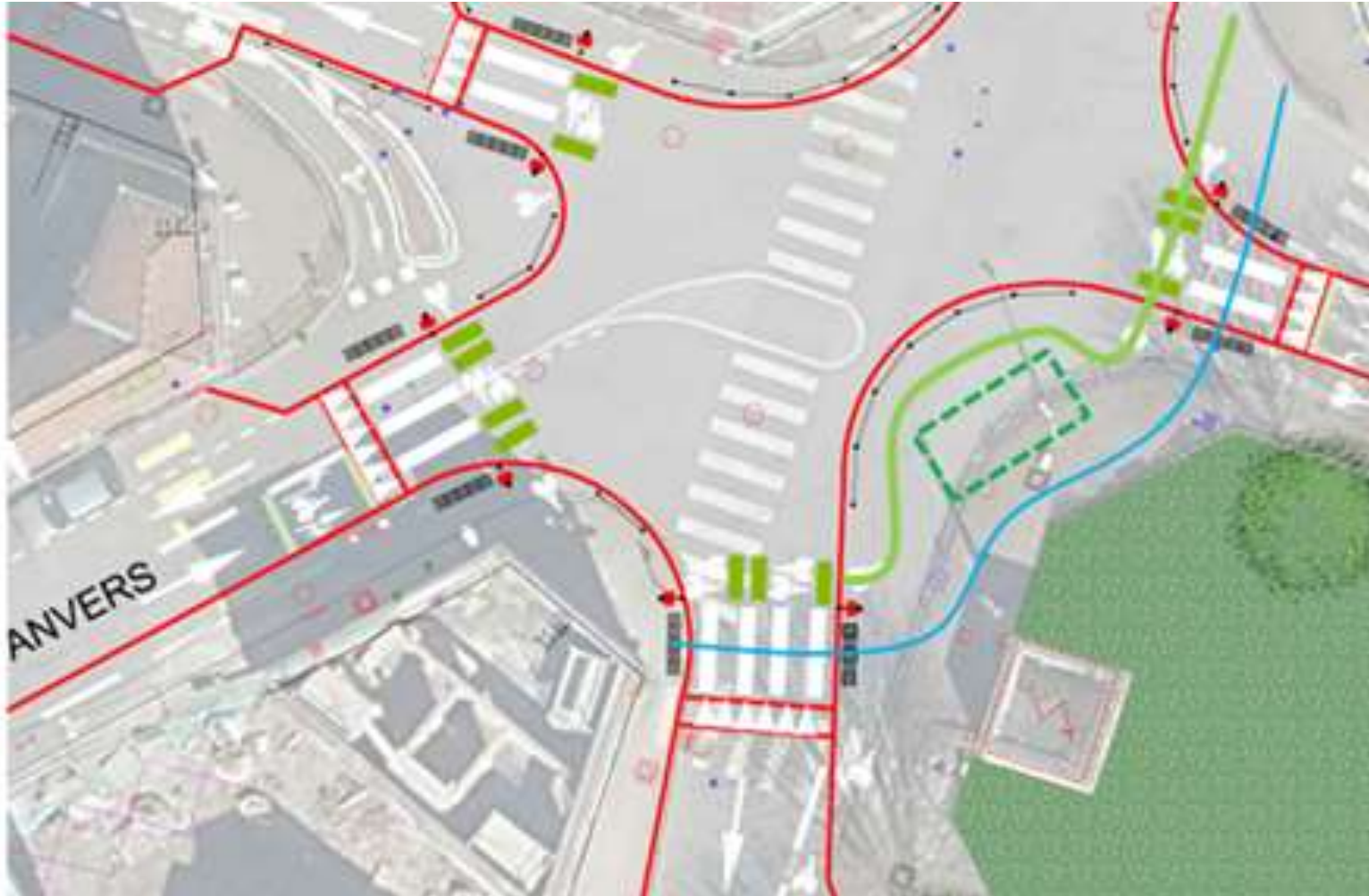
Plan d'étude d'une terrasse déportée
