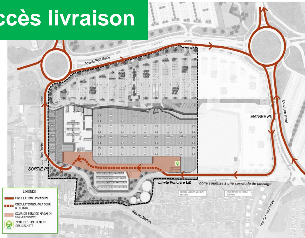
DETAIL DU CIRCUIT LOGISTIQUE DU FUTUR MAGASIN
