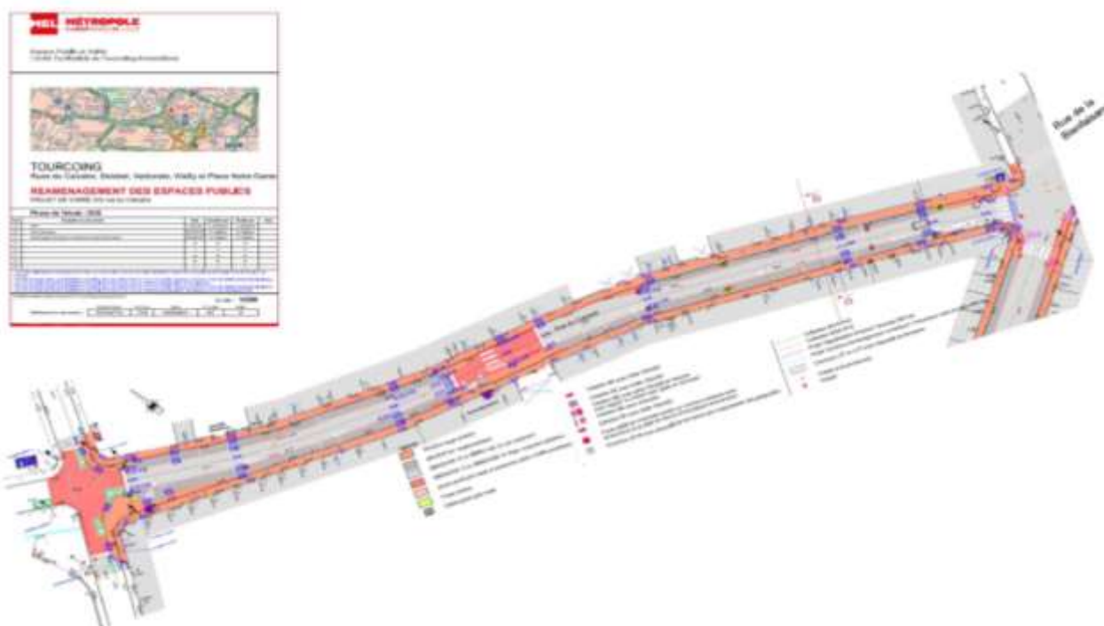
Plan projet
